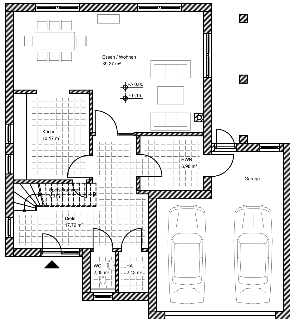
Erdgeschoss
