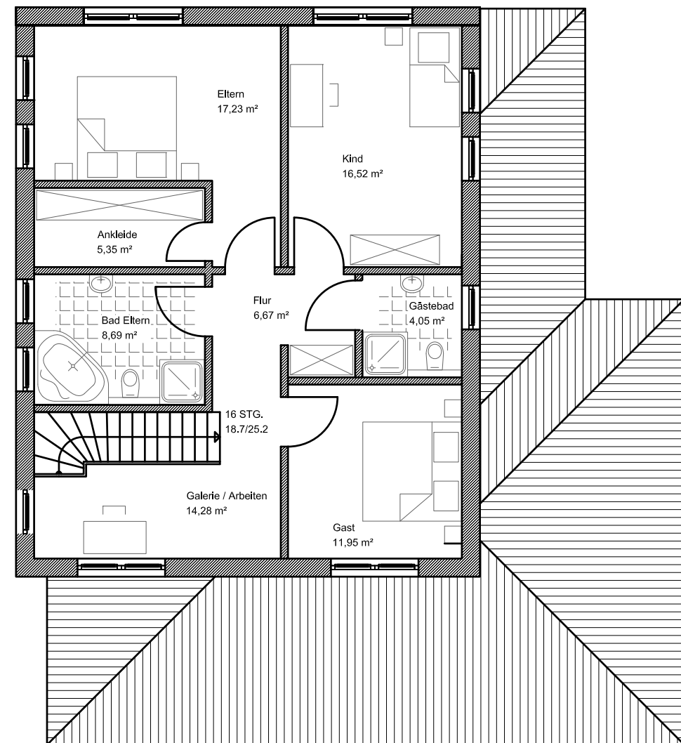
Erdgeschoss
