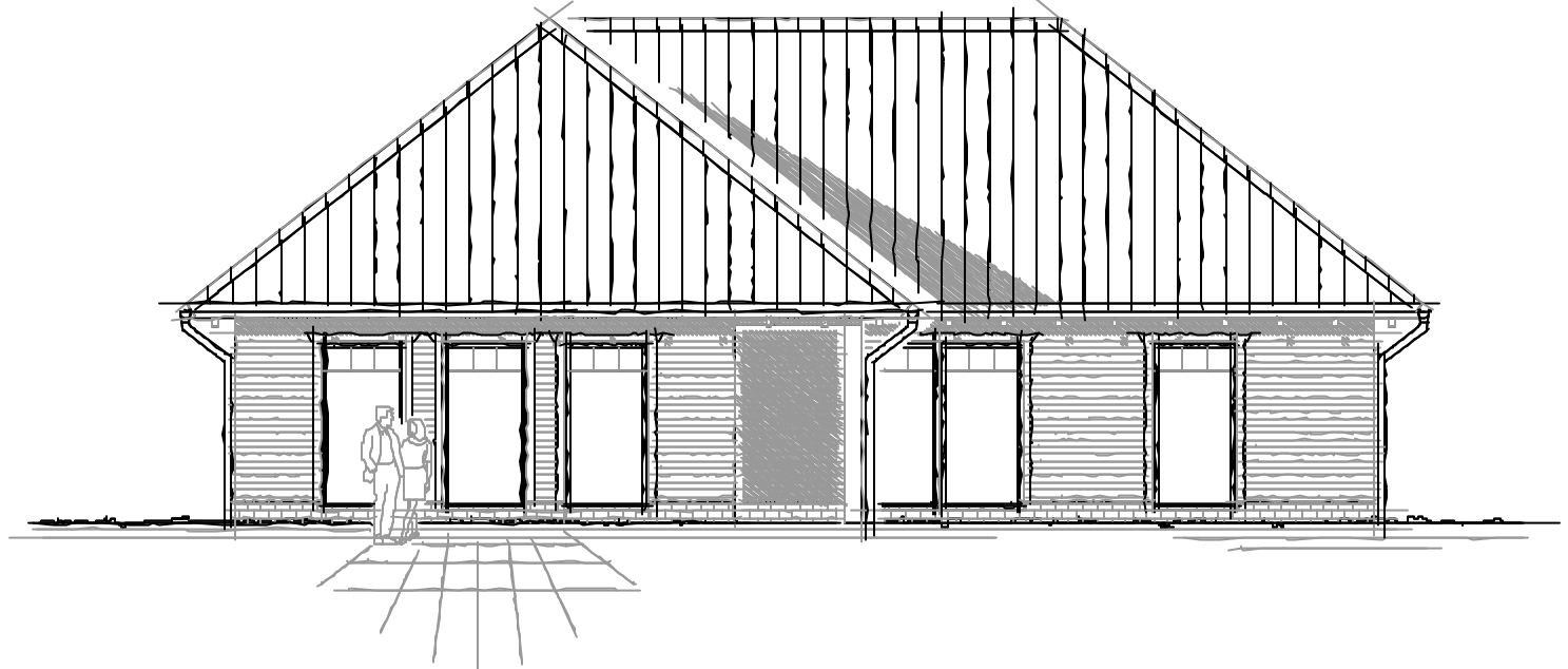
Ansicht Osten
