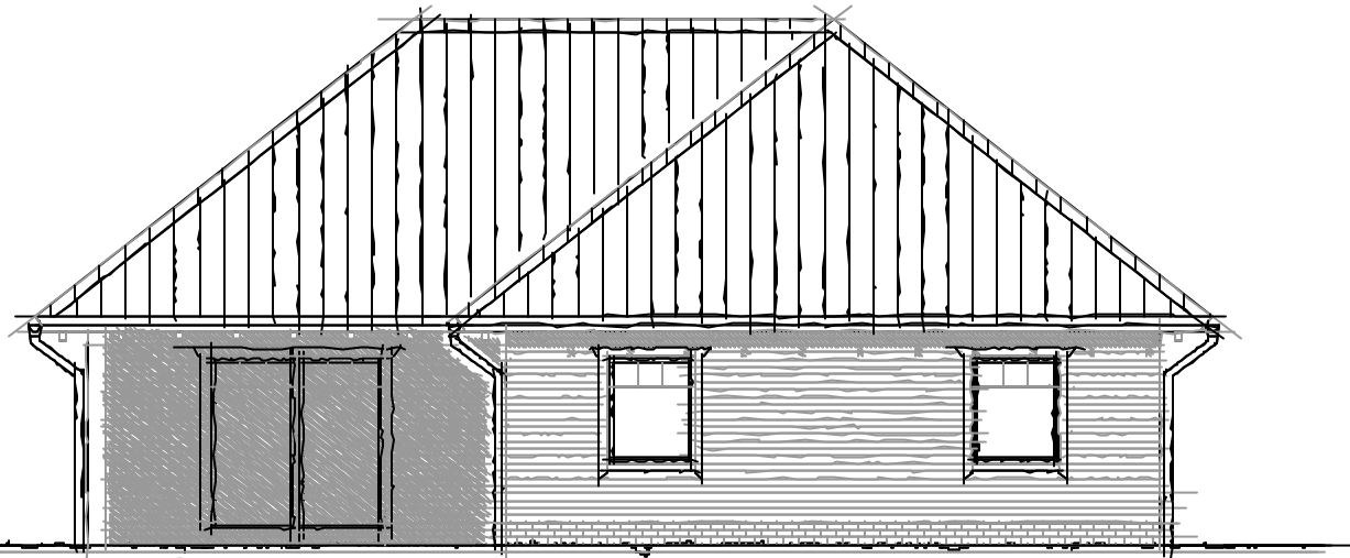
Ansicht Süden
