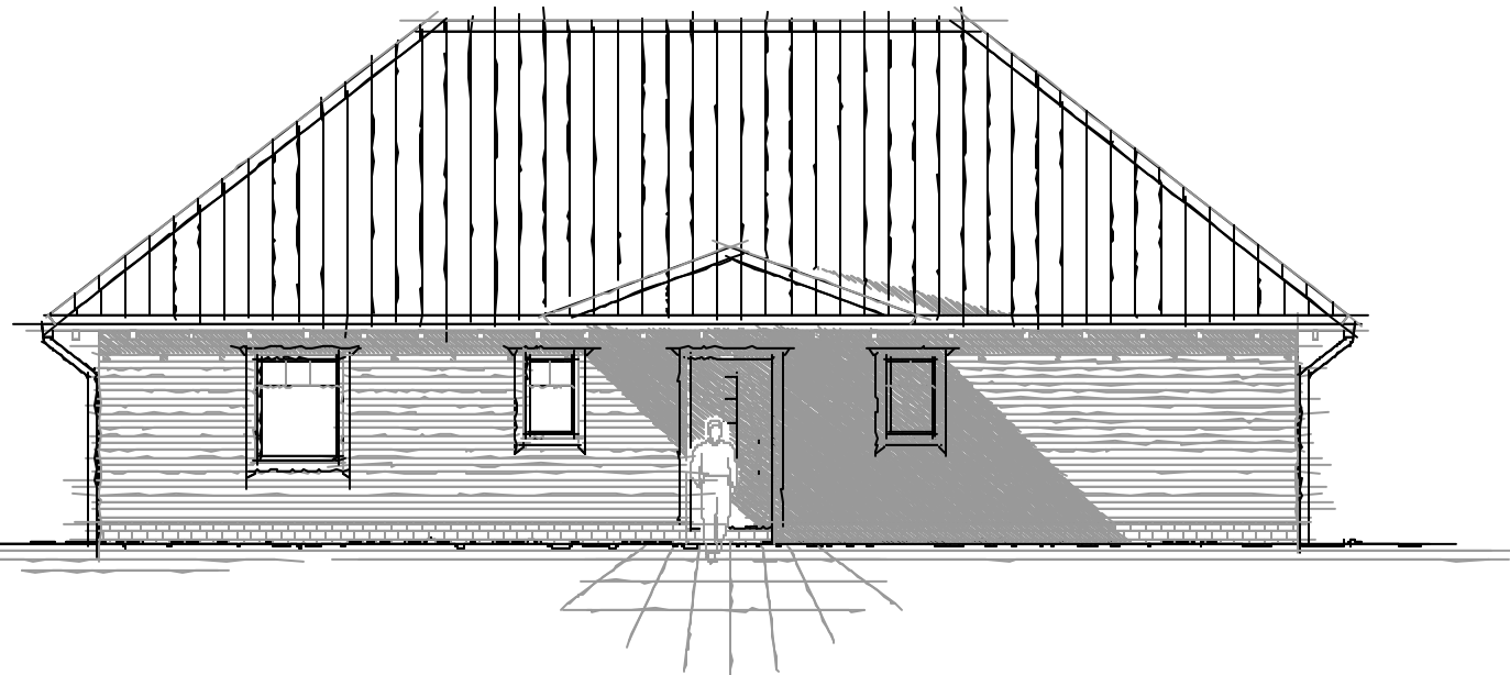
Ansicht Westen
