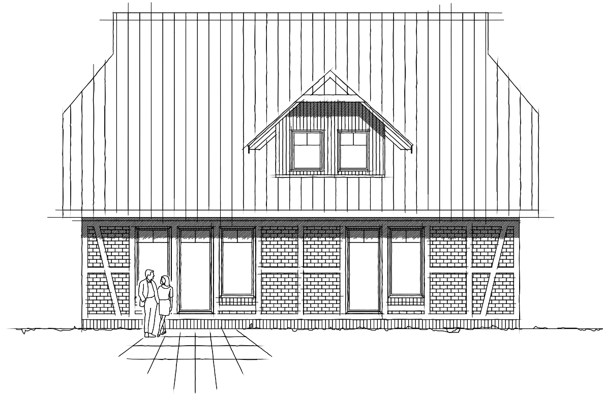
Ansicht Süden
